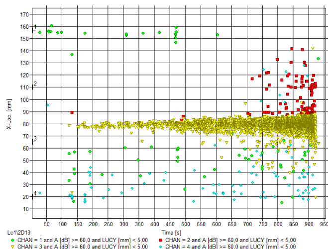
Figura 10. Localización de daño en ensayo 1D.
