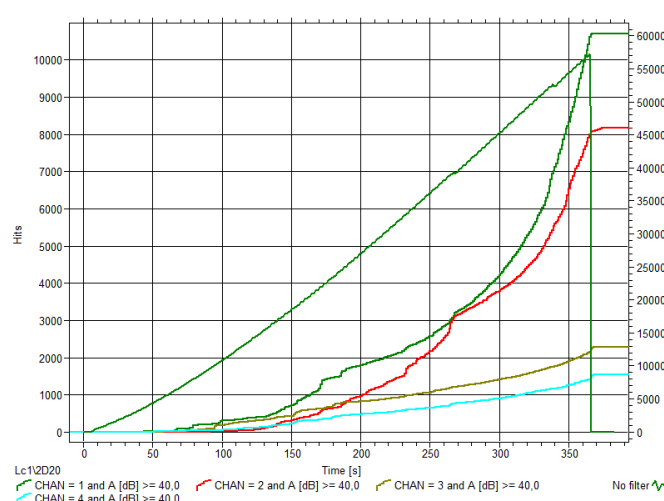
Figura 9. Acumulado de eventos en ensayo 2D.
