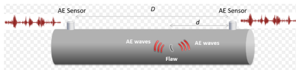
Figura 1. Esquema del principio de propagación de emisiones acústicas (EA).
