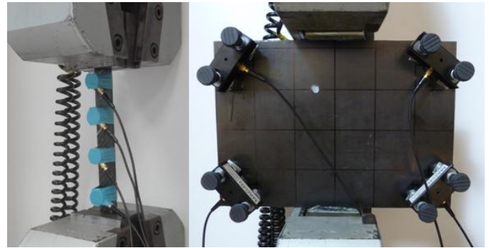
Figura 5. 2 probetas diferentes preparadas para ensayar en máquina de tracción: izq.) (1D), dcha.) (2D).
