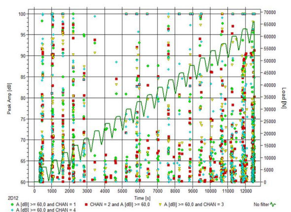
Figura 6. Perfil de aplicación de carga con forma de diente de sierra para evaluación de criterios de daño y eventos acústicos asociados.
